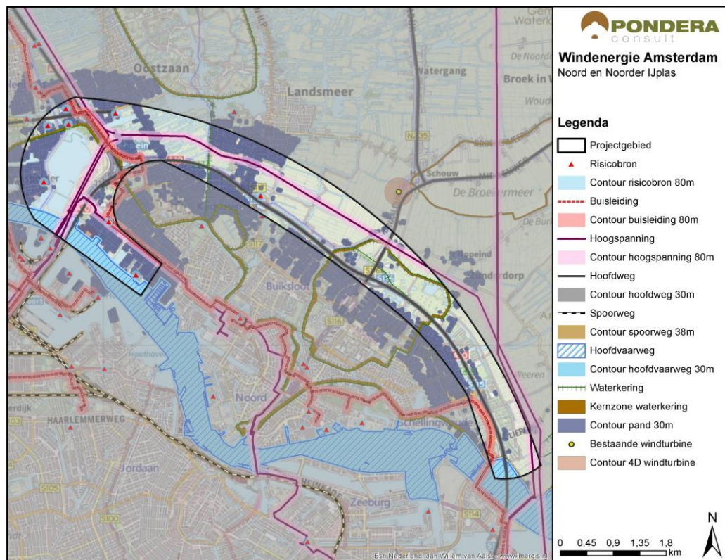
Figuur 2.3 Externe veiligheid & Infrastructuur windturbinecategorie 1
