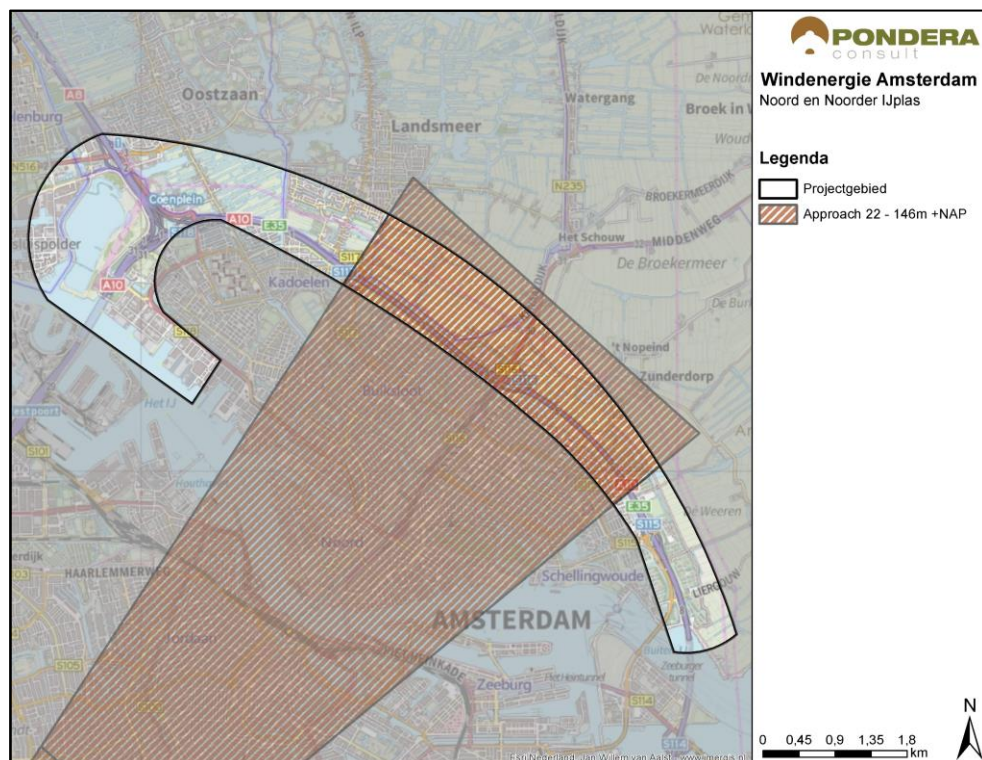
Figuur 2.6 Approach vlak 22 – Luchthavenindelingbesluit Schiphol
