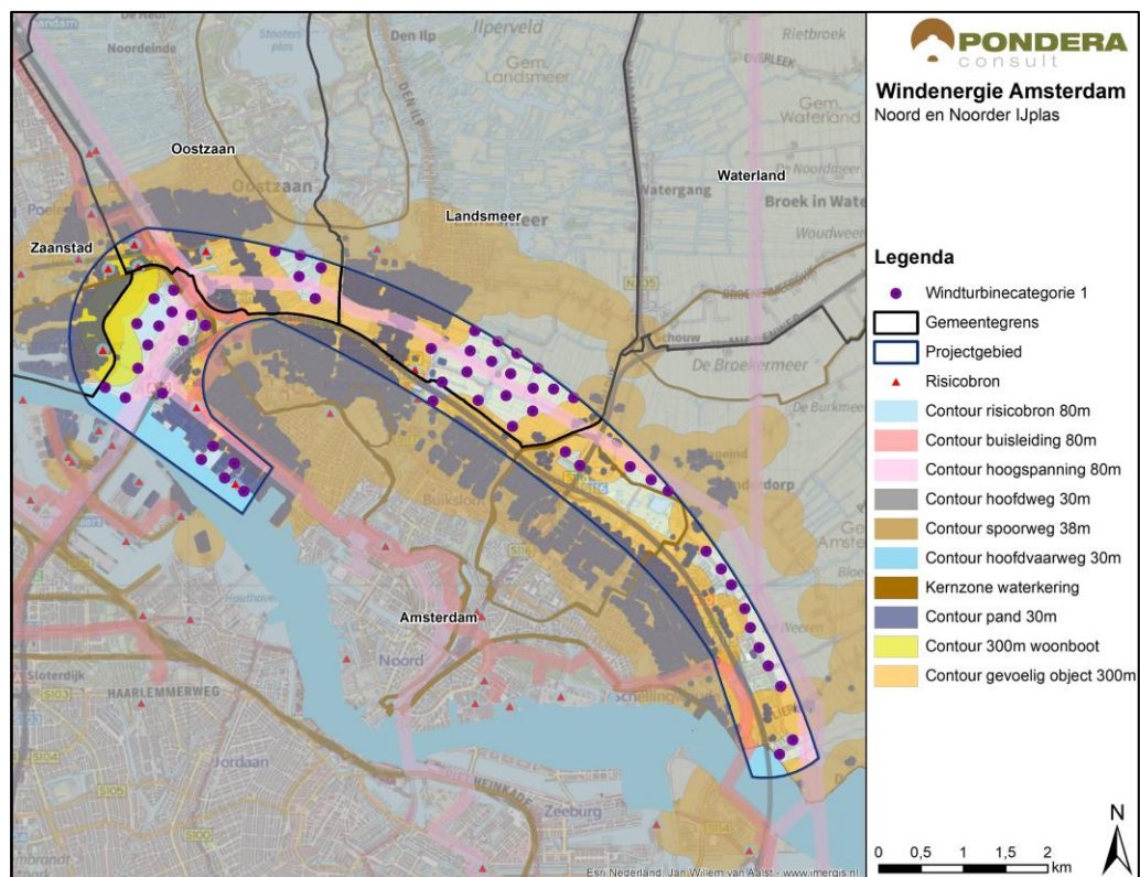
Figuur 3.1 Harde belemmeringen en windturbineposities categorie 1 (56 windturbineposities)
