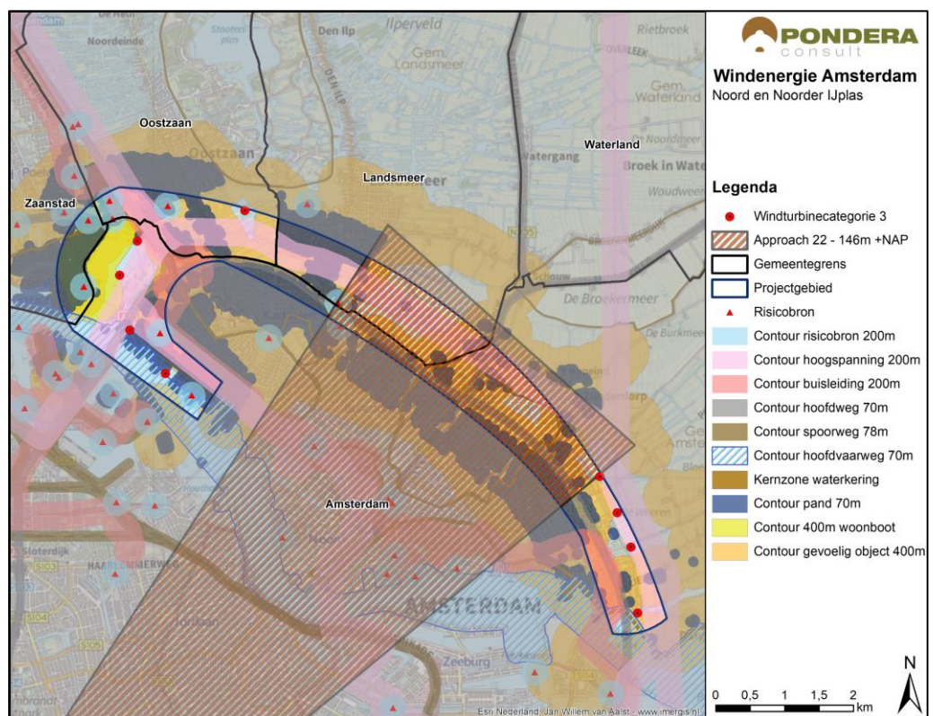
Figuur 3.3 Harde belemmeringen en windturbineposities categorie 3 (9 windturbineposities)
