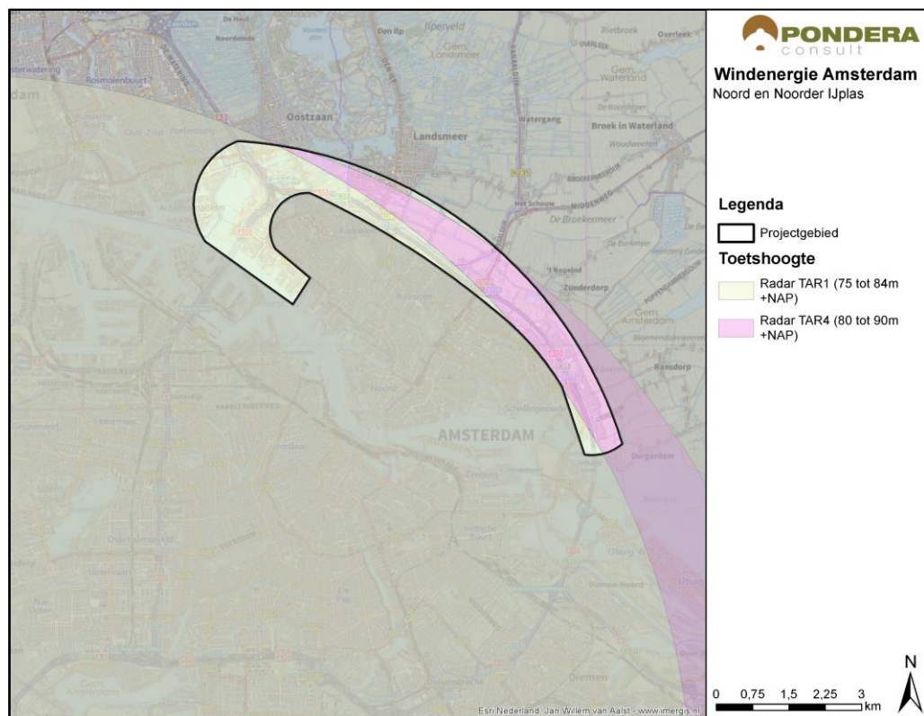
Figuur 2.9 Toetshoogte i.v.m. radar - Luchthavenindelingbesluit Schiphol
