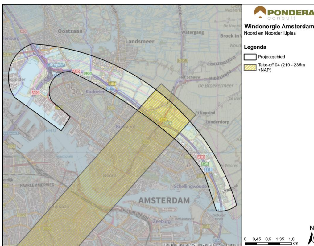
Figuur 2.7 Take-off vlakken 06 en 09 – Luchthavenindelingbesluit Schiphol
