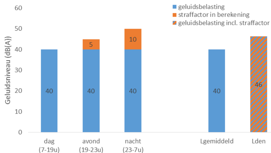
Figuur 4 Berekening L_{den} , met het meetellen van de straffactoren in de avond en nacht.
