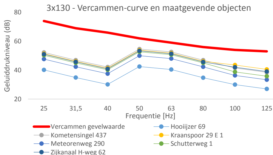
Figuur 23 Vergelijking Vercammen-curve en geluidsdruk niveau maatgevende woningen, 3x130
